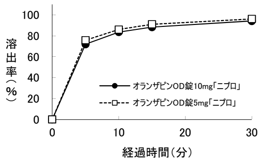
図1-4 試験液:0.2%塩化ナトリウム溶液 (50 rpm)
