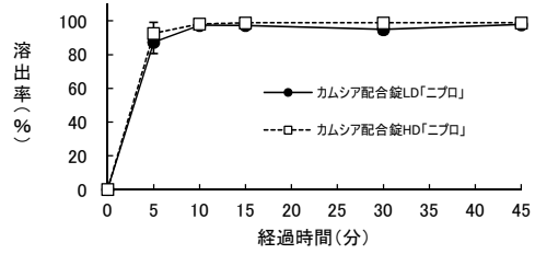
図2-5 試験液:0.2% 塩化ナトリウム溶液 (50 rpm)
