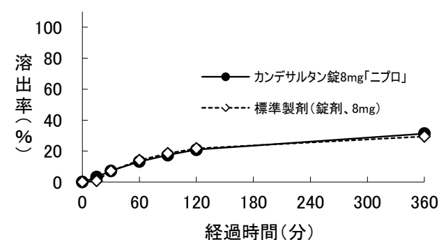
図1-6 試験液:pH 4.0/界面活性剤 (50 rpm)
