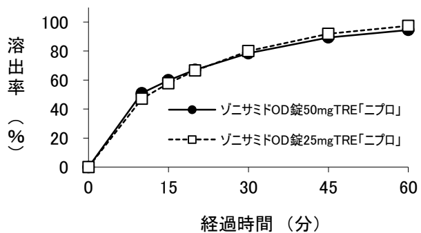
図1-5 試験液:pH 1.2 (パドル法、100 rpm)
