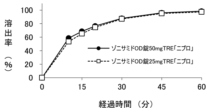
図1-4 試験液:水 (パドル法、50 rpm)
