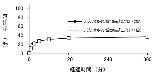
図1-2 試験液:pH 5.0 (パドル法、50 rpm)
