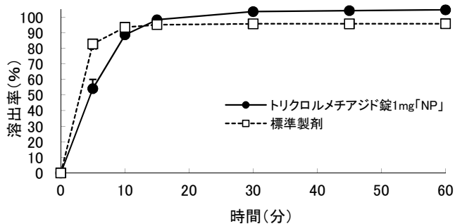
図1-3 試験液pH6.5における平均溶出曲線 (mean±S.D., n=12)
