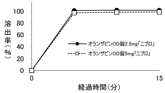
図1-2 試験液:pH 5.0 (50 rpm)
