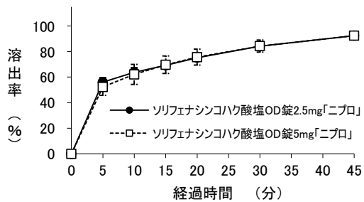
図1-5 試験液: 水 (回転バスケット法、100 rpm)
